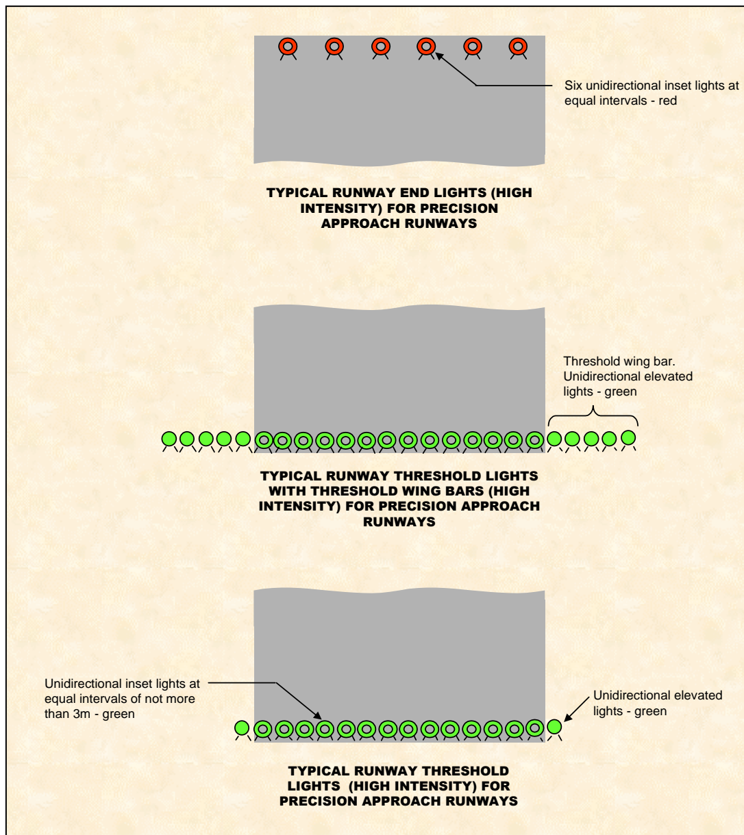
Slika 1.5 Tipična svetla visokog intenziteta praga poletno-sletne staze i svetla visokog intenziteta kraja poletno-sletne staza za precizno prilaznje
